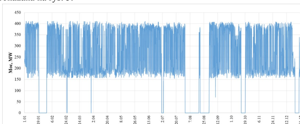
Rys. 3. Typowa praca bloku klasy 450 MW – obecnie (2,1 TWh/r, 4700 h/r)
