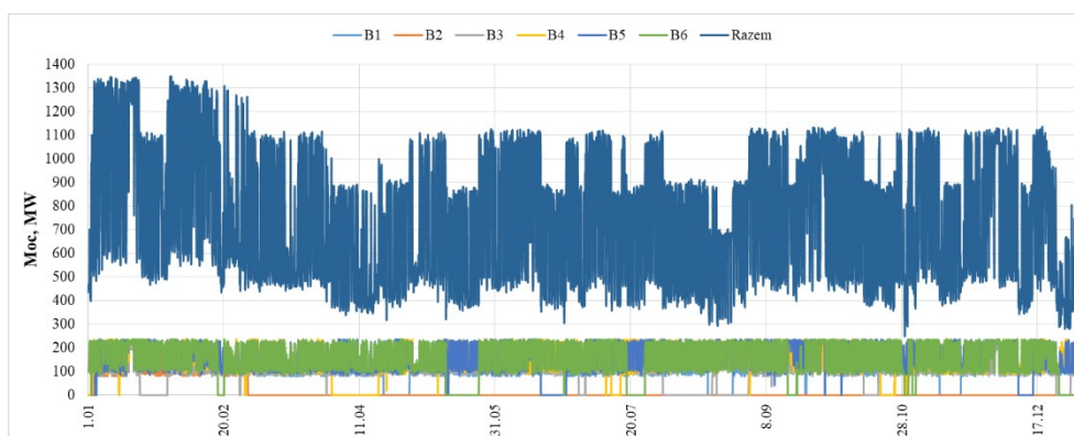
Rys. 6. Praca bloków elektrowni węglowej Turów (2017 r)
