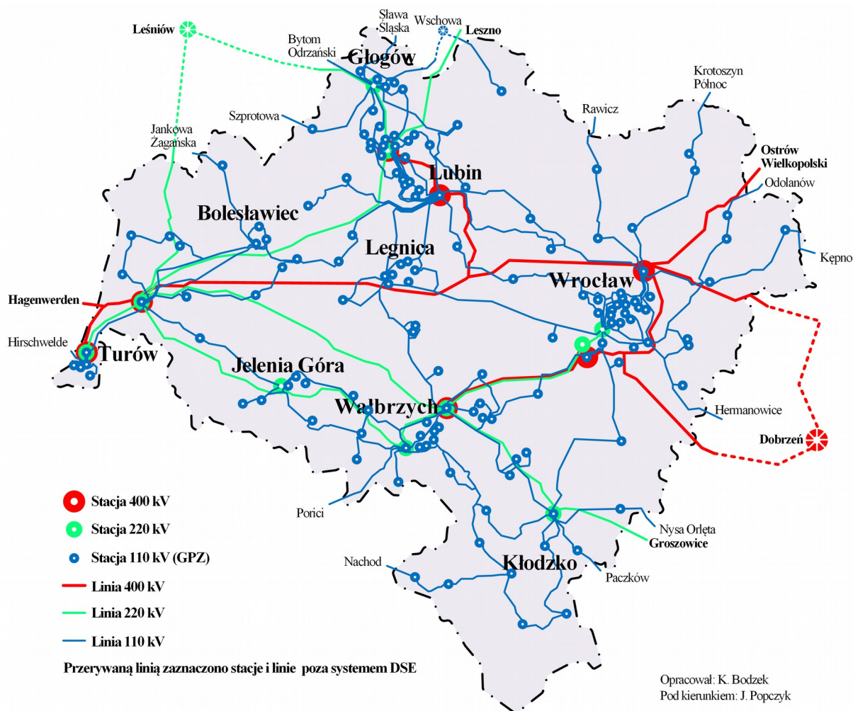
Rys. 9. Mapa pogładowa sieci zasilającej województwa dolnośląskiego
