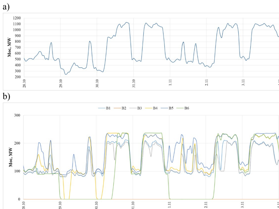
Rys. 8. Elektrownia Turów a) sumaryczna produkcja, b) praca poszczególnych bloków (28.10.2017 – 4.11.2017)
